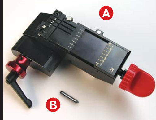
A. Mord.Cifrado/Grabado-R1/R12 (cód. D734232ZB) B. Fresa - W146 (cód. D734267ZB)
